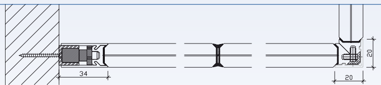
HORIZONTALSCHNITT FIXVERGLASUNG
