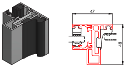
Basis-G Zargenprofil für Glasanschluss
